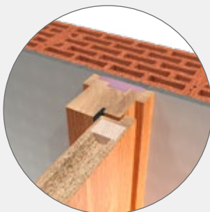
RAHMENSTOCK Türblatt furniert
