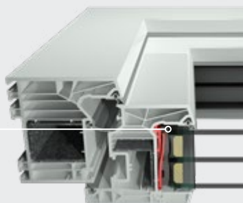
Seitenansicht Rahmen/Flügel
