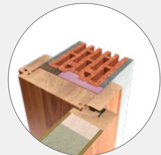
BRANDSCHUTZTÜR Doppelfalz mit Überschlagsdichtung
