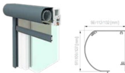
VORO ZIP BRAVO
