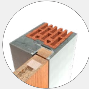
AGS ZARGE Türblatt furniert | Flächenbündig nicht in die Leibung öffnend
