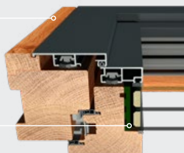
Seitenansicht Rahmen/Flügel
