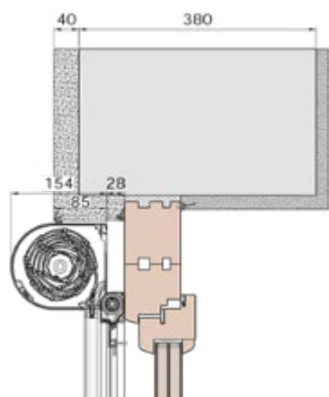
Mit Stockaufdoppelung VORO BRAVO mit kombiniertem Insektenschutz-Rollo
