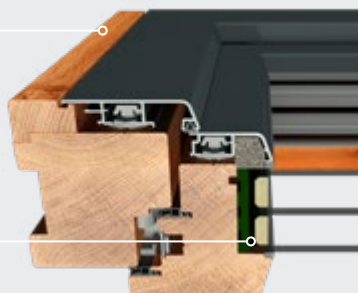
Seitenansicht Rahmen/Flügel
