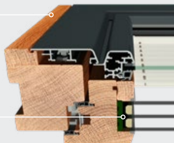
Seitenansicht Rahmen/Flügel
