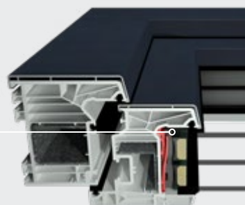
Seitenansicht Rahmen/Flügel
