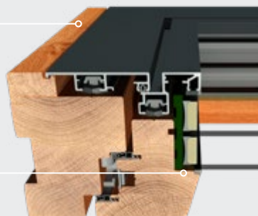
Seitenansicht Rahmen/Flügel
