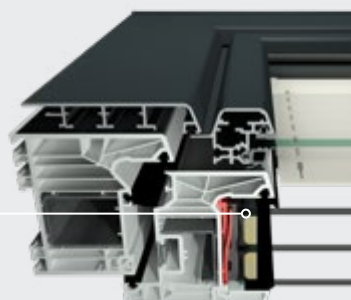
Seitenansicht Rahmen/Flügel
