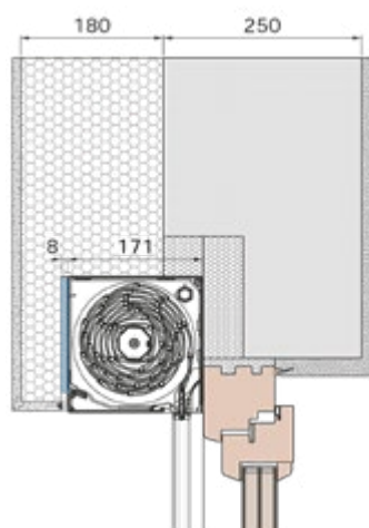
Mit Wärmedämmverbundsystem VORO SICHT 90 WDVS
