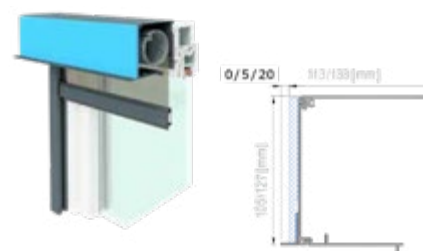
VORO ZIP PUTZ-90
