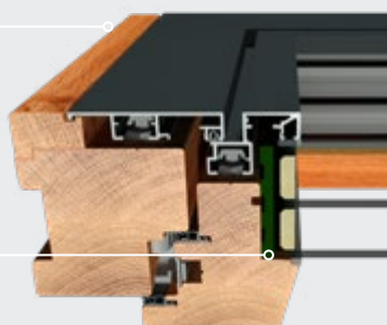
Seitenansicht Rahmen/Flügel
